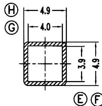
A-A SECTION
