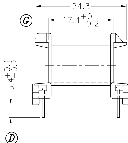
SEC.A-A
