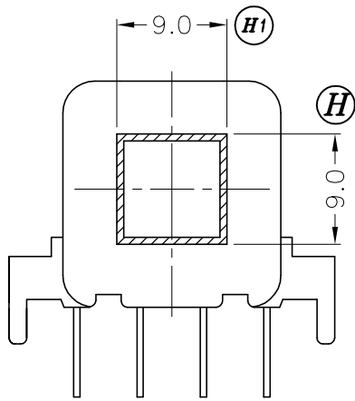
SEC. A-A
